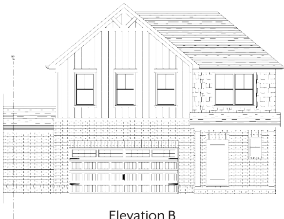
Elevation B
